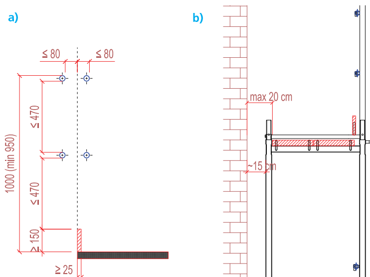
Rys. 12. Balustrada na rusztowaniu: a) rozmieszczenie elementów – wymiary w mm, b) dopuszczalna odległość od ściany bez konieczności stosowania balustrad wewnętrznych.
